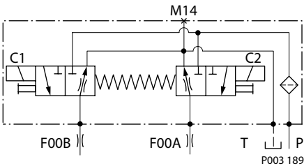
FNR-原理图
