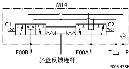
EDC-原理图
