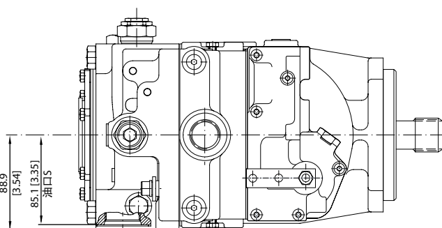
"Y"视图
