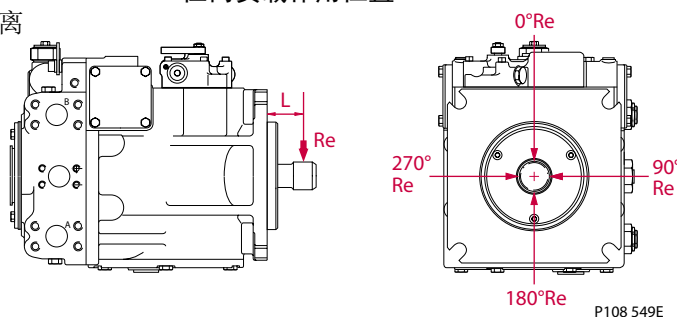
径向负载作用位置
