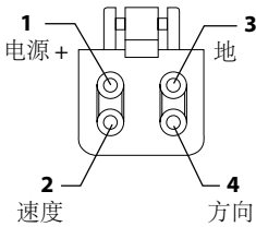
4 针Deutsch® Plug DT 系列电气接头
