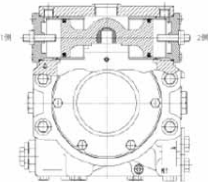
排量限制器
