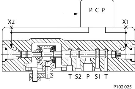
剖视图
