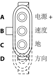
3 或4 针Delphi 电气接头
